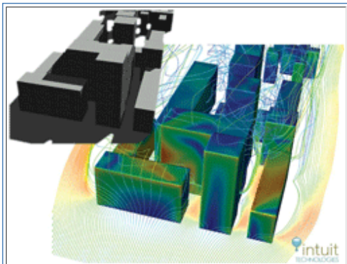
Modélisation CAO du bâtiment et du résultat final des pertes thermiques (trajectoires de l'air colorées par la vitesse du "vent") Intuit Technologies © Tous droits réservés
